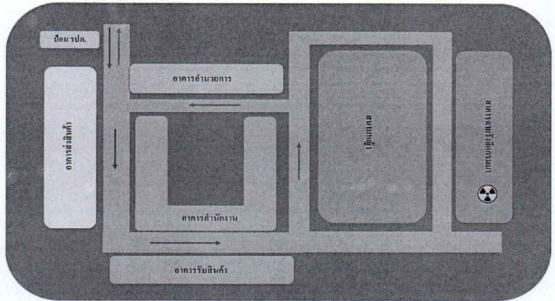
ภาพที่ ๑ แสดงแผนผังภายในสถานประกอบการทางรังสี
