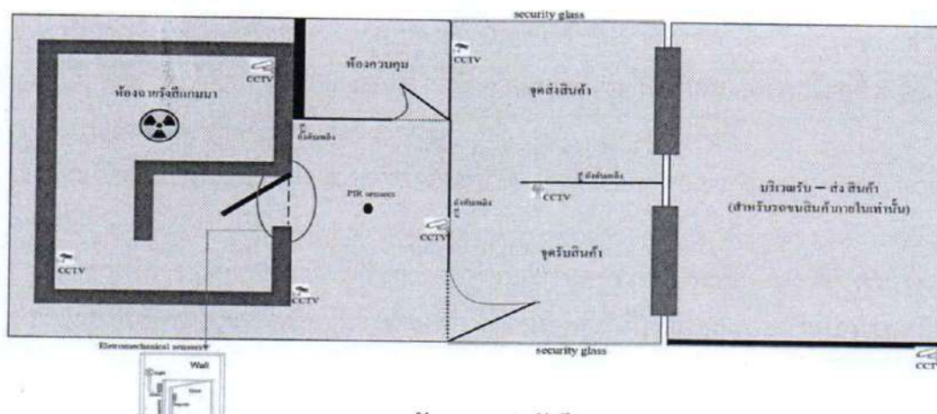
ผังอาคารฉายรังสีแกมมา
